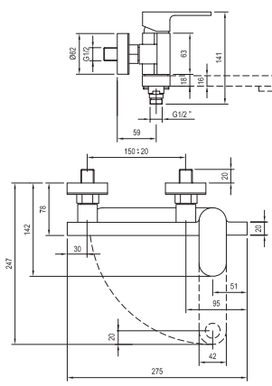
Vanová nástěnná baterie bez setu
