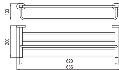
Police na ručníky s držákem, 66 cm CR 330.00
