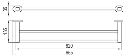
Držák na ručník CR 320.00
