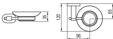
Držák s mýdlenkou CR 200.00
