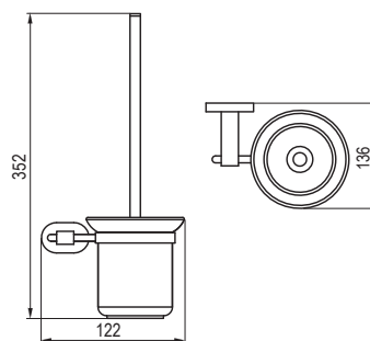
Držák s nádobkou a WC štětkou CR 410.00
