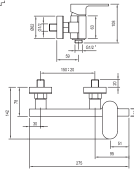
Sprchová nástěnná baterie bez setu
