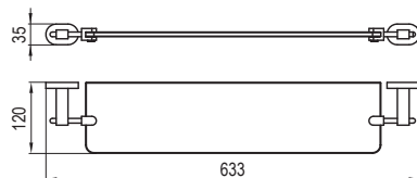
Polička skleněná 64 cm CR 500.00
