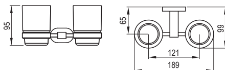
Držák se dvěma pohárky CR 220.00
