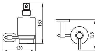
Dávkovač na mýdlo CR 230.00
