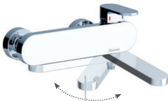
Vanová nástěnná baterie s otočným ramínkem bez setu 150 mm CR 022.00/150
