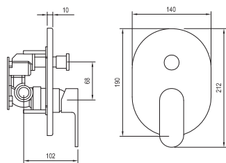
Podomítková baterie s přepínačem
