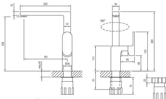
Dřezová stojánková baterie
