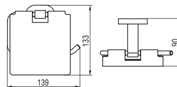
Držák na WC papír CR 400.00
