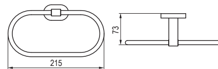
Držák na ručník oválný CR 300.00
