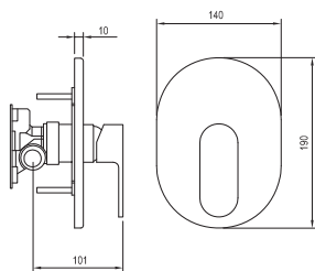
Podomítková baterie bez přepínače
